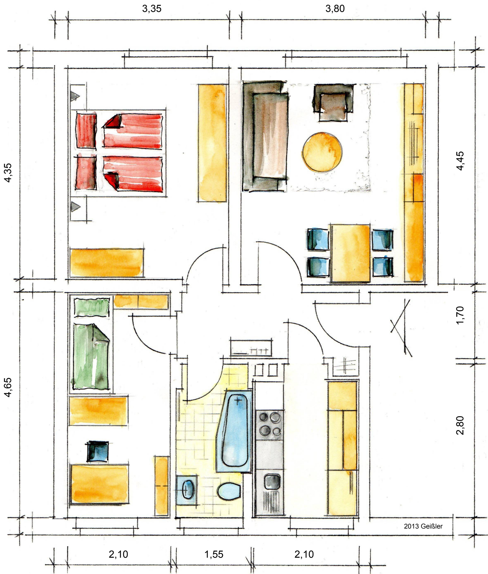
3- Raum linke Wohnung Schulstraße 30/32
